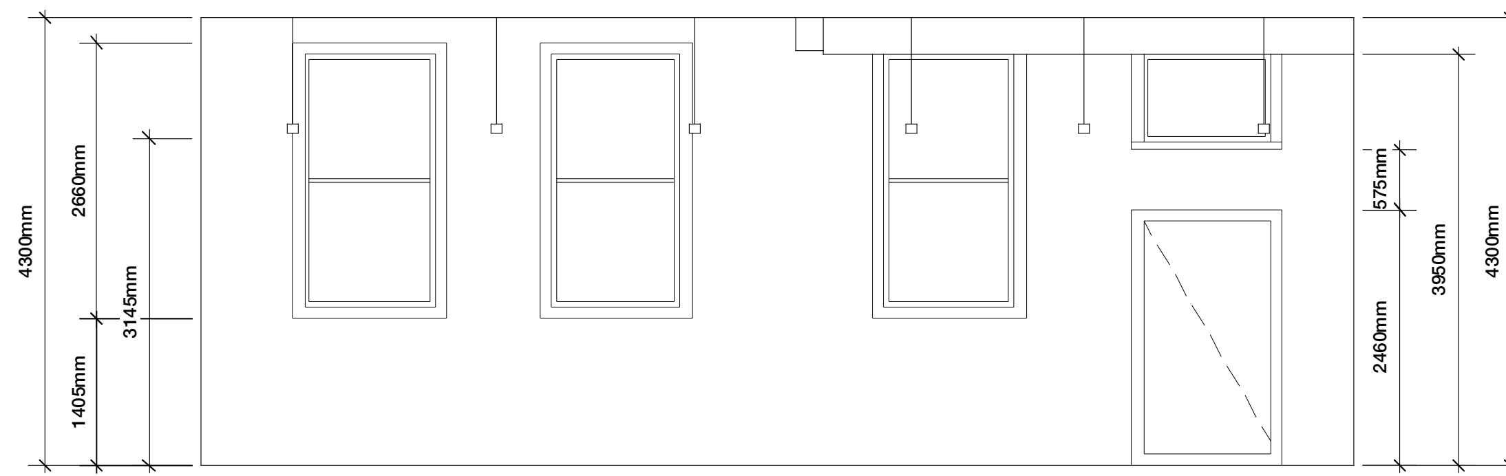
ELEVATION A
